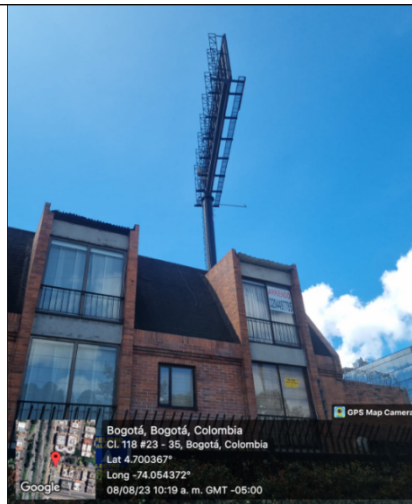
Foto 2. Vista de la estructura de la valla
